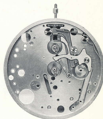
Mécanisme 1 fonction
